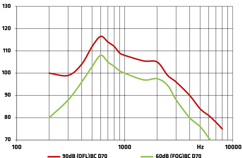
dB OFL90 Ausgangskraftpegel, FOG(60) akusto-mechanischer Kraftpegel
